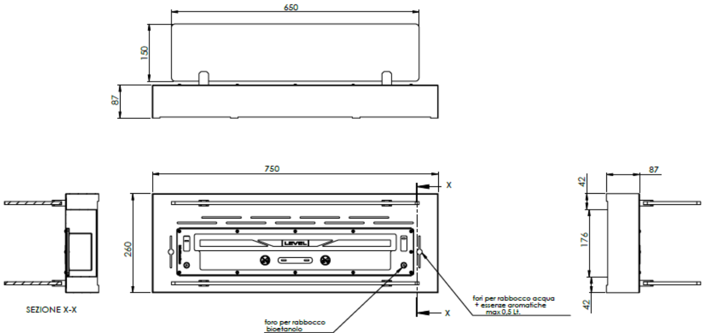
Desenho técnico do suporte para o queimador BR600R
